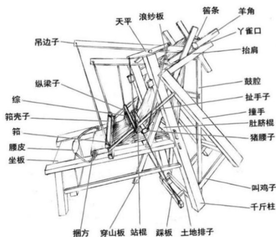
图1 近代夏布腰机结构标注图
